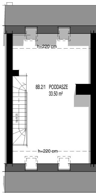
PODDASZE
