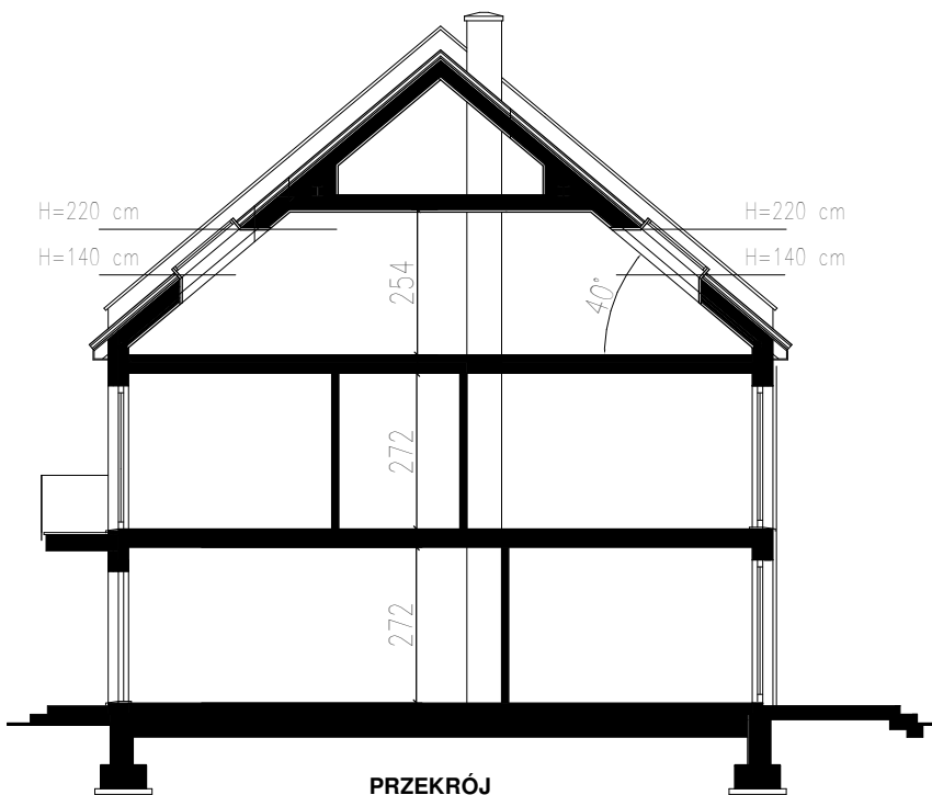
PRZEKRÓJ
